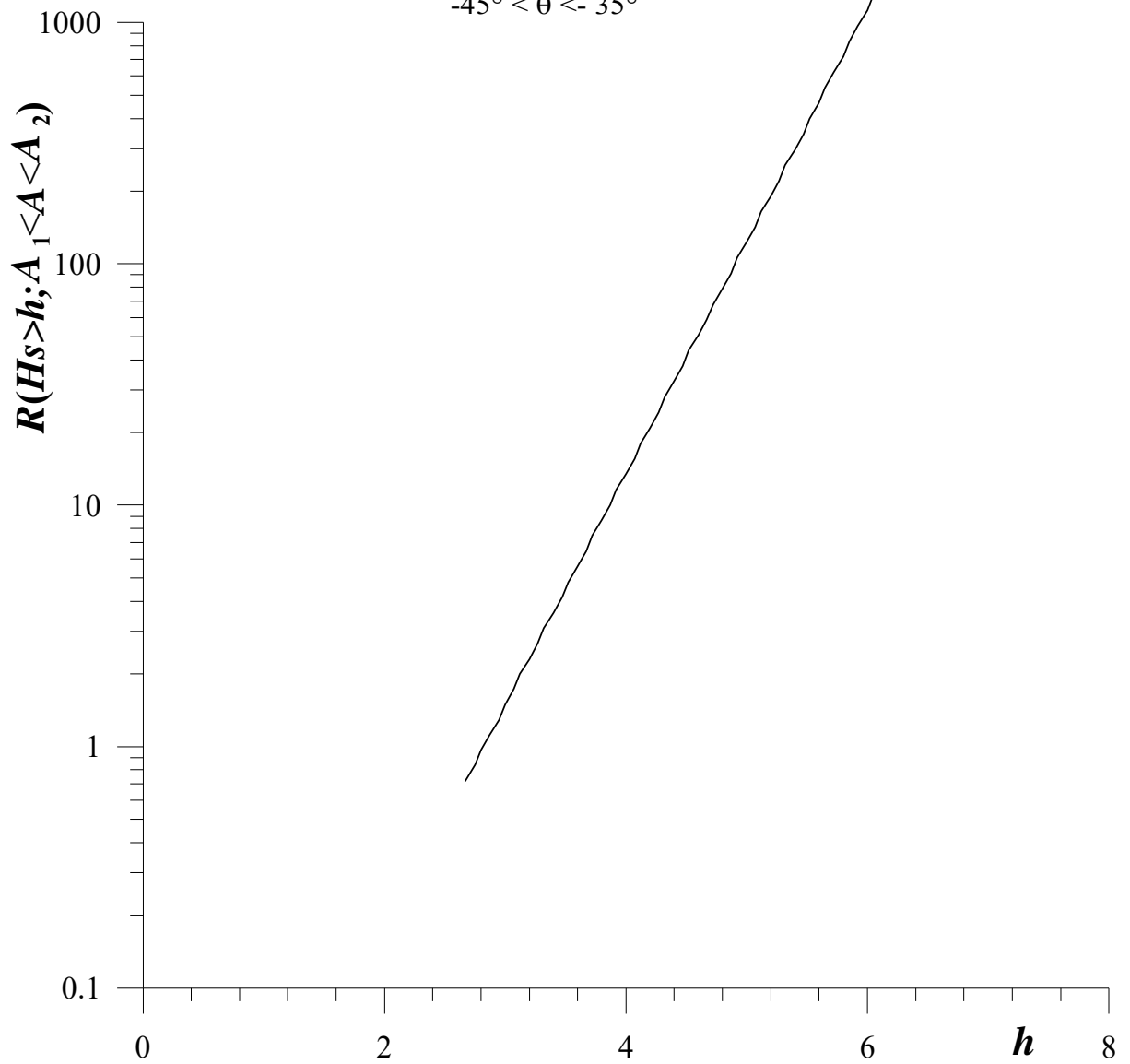
Fig. 6.1e – Periodo di ritorno R(H_s > h; \theta_1 < \theta < \theta_2) di mareggiate nelle quali la H_s superi una qualsiasi assegnata soglia h e la direzione di propagazione delle onde \theta sia compresa entro assegnati settori (\theta_1, \theta_2) .
