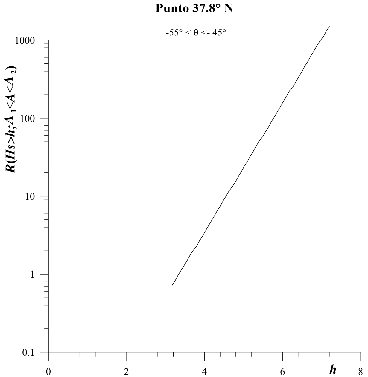
Fig. 6.1d – Periodo di ritorno R(H_s > h; \theta_1 < \theta < \theta_2) di mareggiate nelle quali la H_s superi una qualsiasi assegnata soglia h e la direzione di propagazione delle onde \theta sia compresa entro assegnati settori (\theta_1, \theta_2) .
