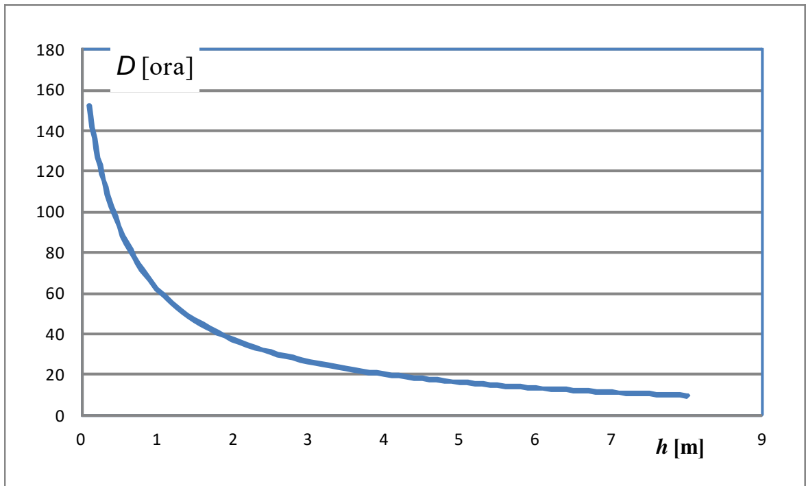
Fig. 7.2. Durata media \bar{D} , dell'altezza significativa h .
