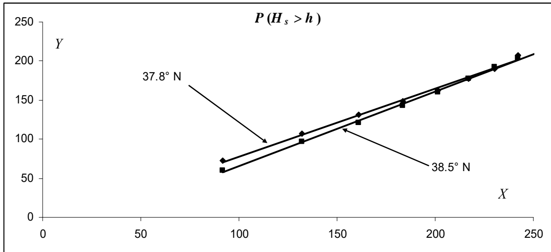
Fig. 3.1 – Confronto tra le probabilità di superamento della H_s nel punto 37.8° N e nel punto 38.5° N.
