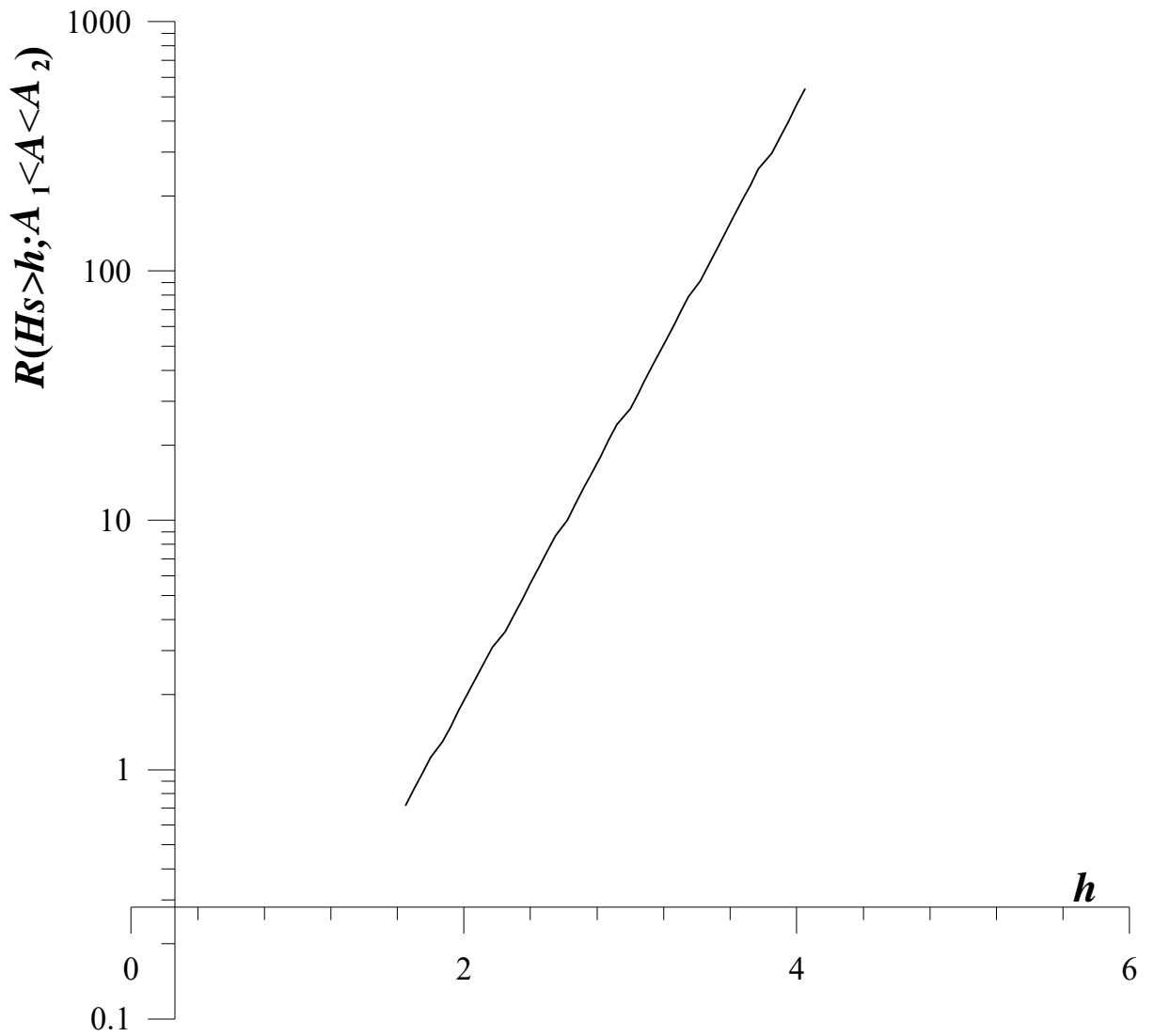
Fig. 6.1h – Periodo di ritorno R(H_s > h; \theta_1 < \theta < \theta_2) di mareggiate nelle quali la H_s superi una qualsiasi assegnata soglia h e la direzione di propagazione delle onde \theta sia compresa entro assegnati settori (\theta_1, \theta_2) .
