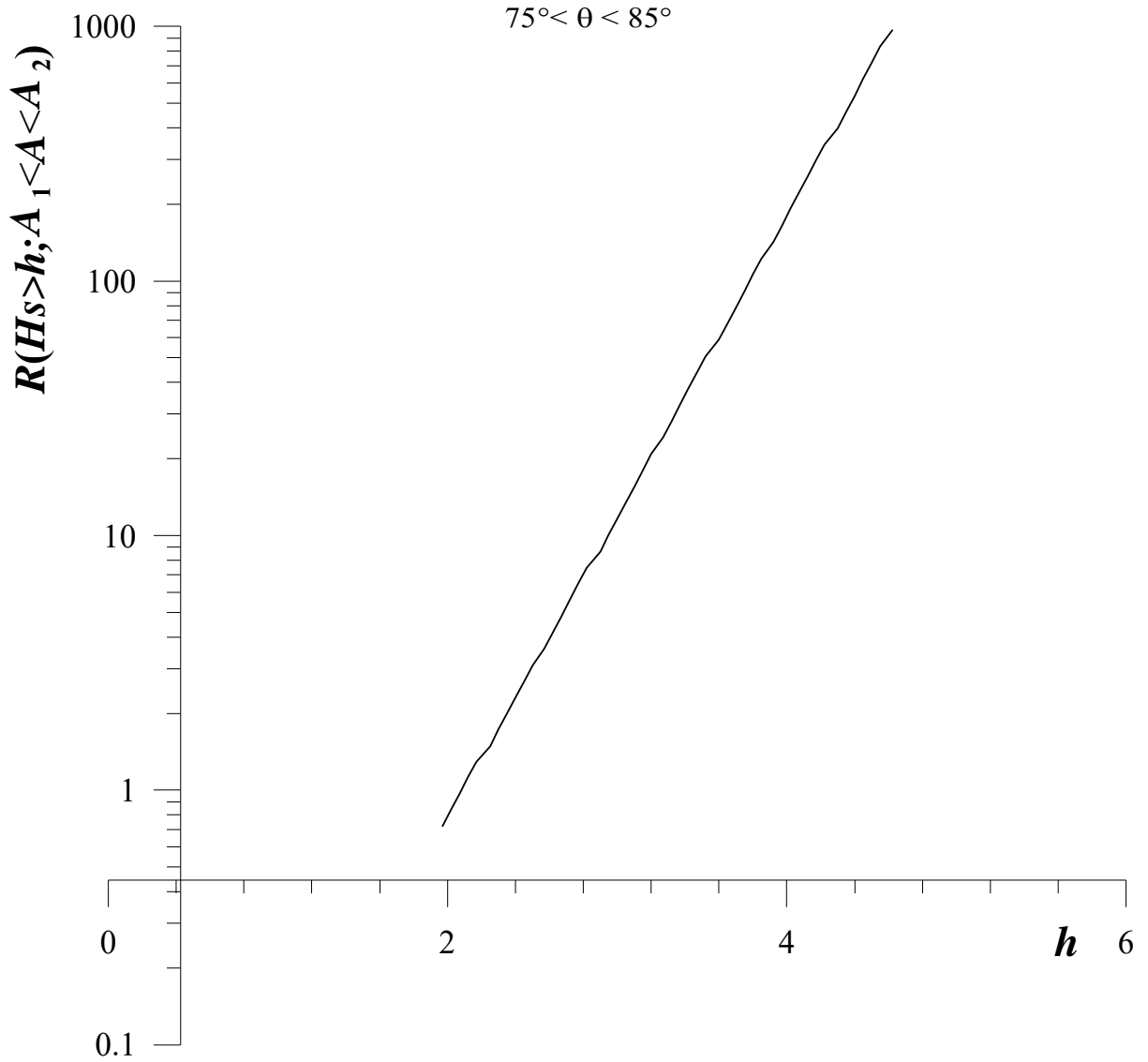
Fig. 6.1n – Periodo di ritorno R(H_s > h; \theta_1 < \theta < \theta_2) di mareggiate nelle quali la H_s superi una qualsiasi assegnata soglia h e la direzione di propagazione delle onde \theta sia compresa entro assegnati settori (\theta_1, \theta_2) .
