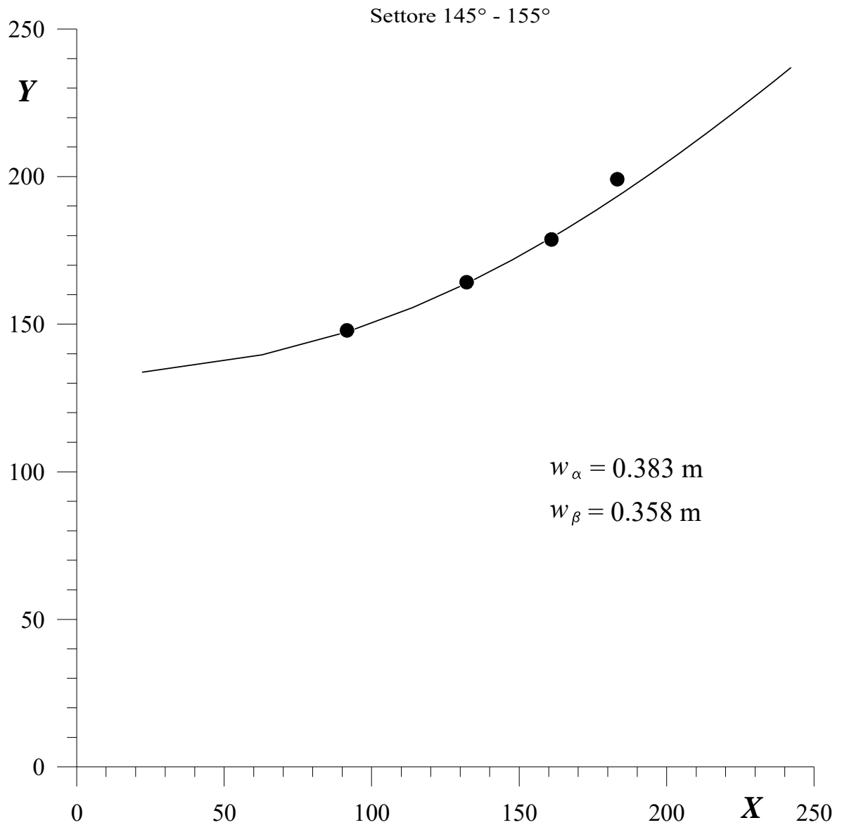
Fig. 4.2.i – Punto [37.8°N-15.5°E]: probabilità di superamento direzionale. Il piano della rappresentazione è quello delle variabili ausiliarie X e Y definite dalla (1). [Nota: La probabilità di superamento per il presente settore è stata ottenuta per interpolazione tra i valori di probabilità dei settori contigui (325° - 335° e 345°-355°) in quanto il dato ondometrico risultava incerto e di difficile interpretazione.]
